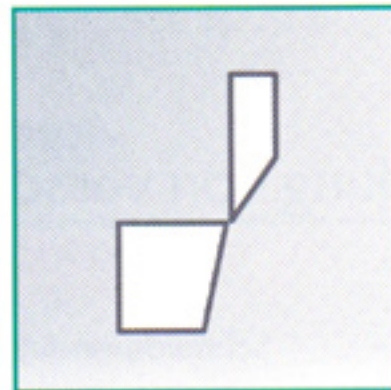
Scherschnitt
